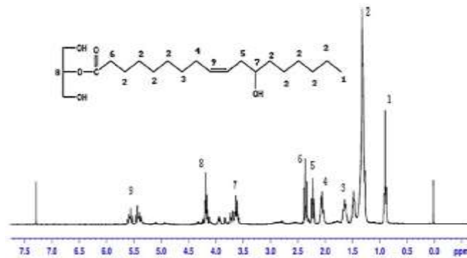
Fig. 5. 1 H NMR spectra of GCO.
