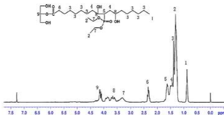
Fig. 7. 1 H NMR spectra of POFPL.tif.
