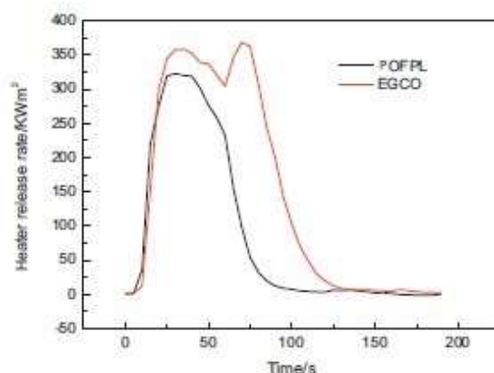
Fig. 12. HRR curves for GCO filled PU foam, POFPL filled PU foam.
