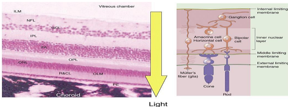
fig.2 Retina
